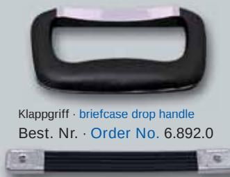
Riemengriff · strap handle Best. Nr. · Order No. 6.894.0
